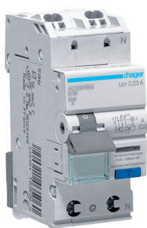
ADS917D
